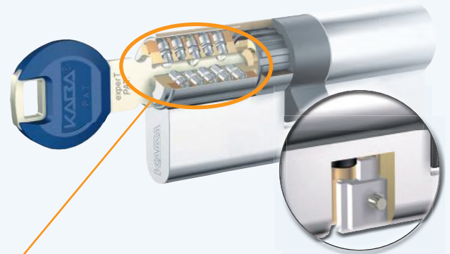
4 radial angeordnete Stiftreihen
